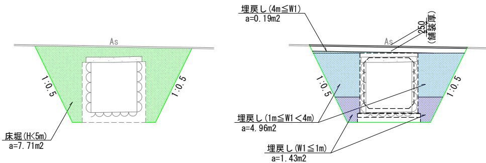
(床堀)
