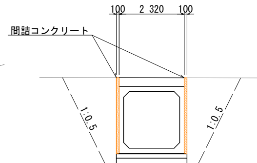
(上流側断面)
